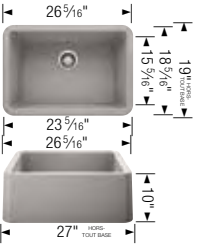
Éviers IKON MD :
