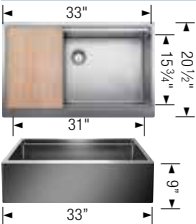
QUATRUS MD R15 U 2 TABLEAU AVANT EXPOSÉ
