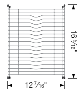
Panier à vaisselle flottant 406999
